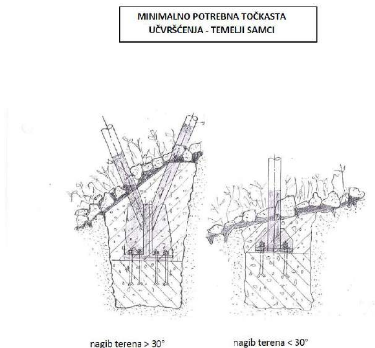
Slika 11 - prikaz mogućeg načina temeljenja
