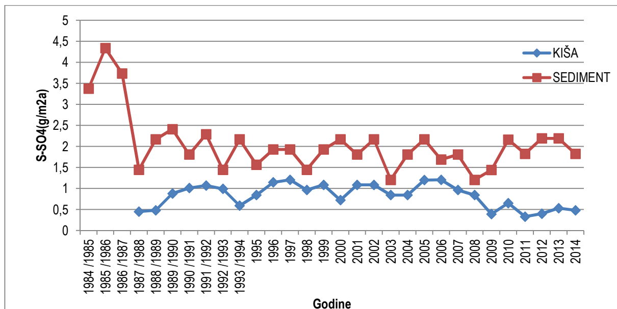
Slika 88: Taložanje sumpora u obliku sulfata ( S-SO_4^{2-} ) u taložnoj tvari (sedimentu) i kišnici
